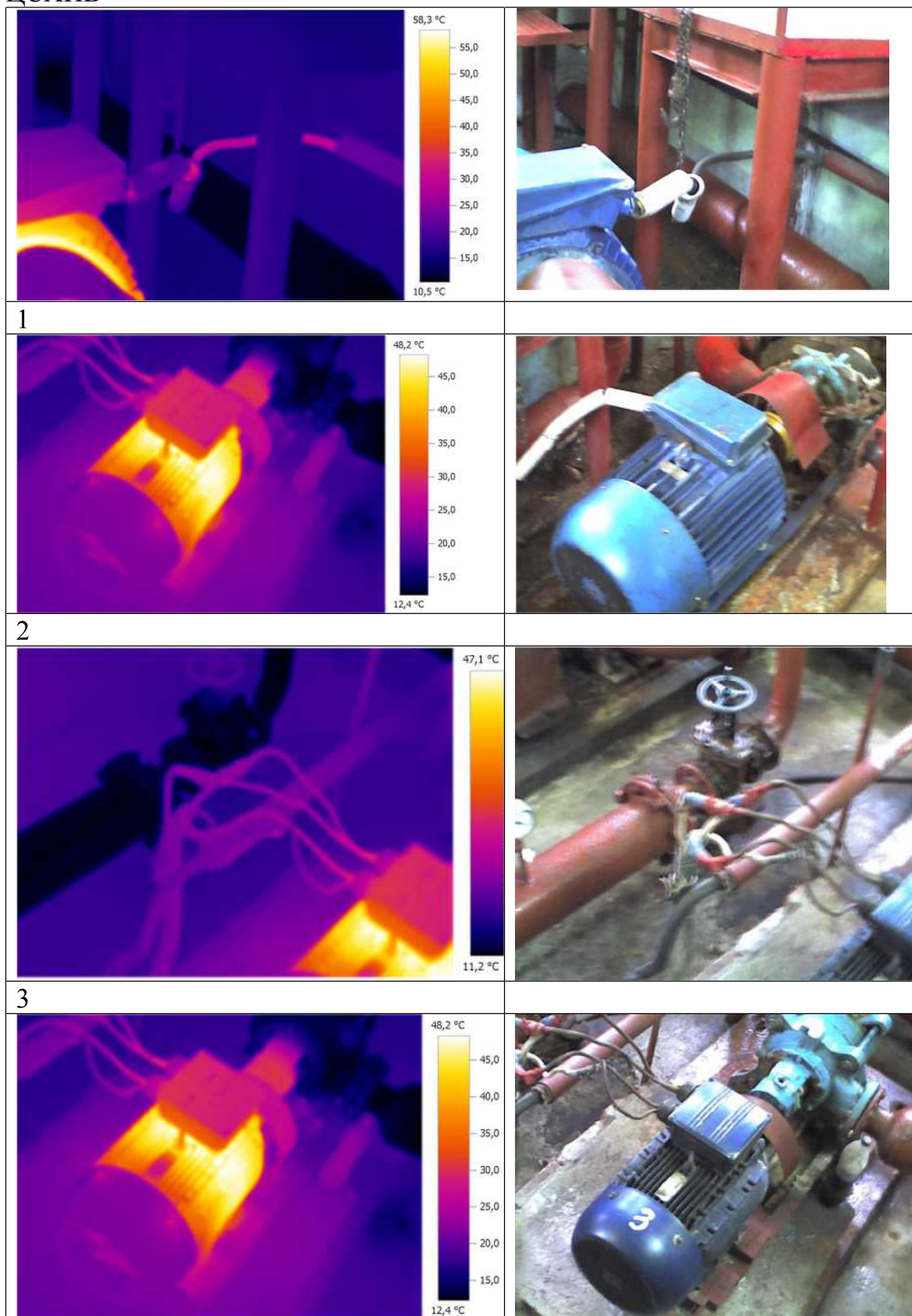
Рисунок 11 Тепловизионное (термографическое) обследование объектов ЦСХПВ
