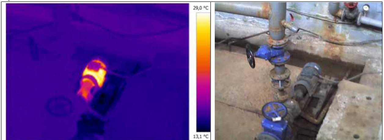
Рисунок 15 Тепловизионное (термографическое) обследование объектов ЦСХПВ
