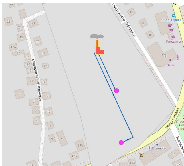
Рисунок 24 Схема теплоснабжения котельной № 8
